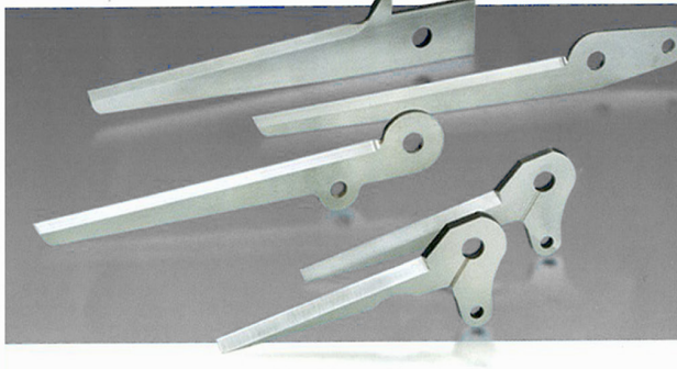
Cuchillas de corte y anillos tensores
